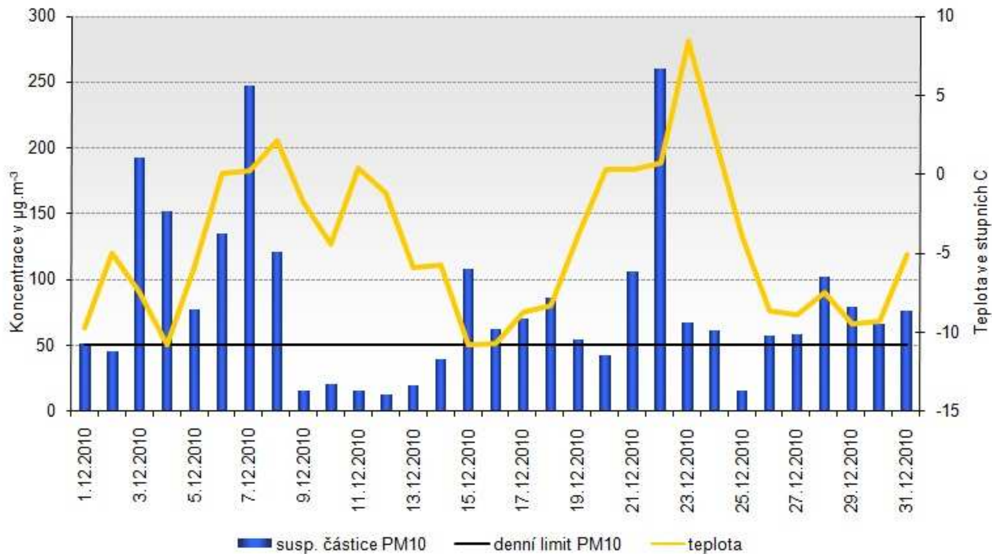
Průměrné denní koncentrace částic PM 10 a průměrná denní teplota na AMS Orlová, 2010
